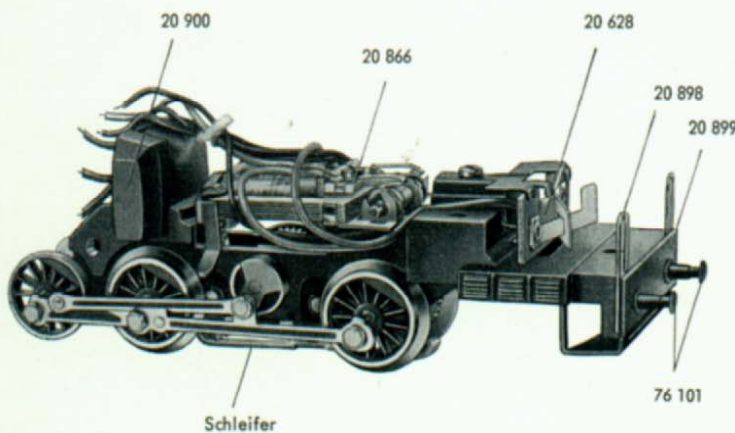
Fig. 4a Treibgestell (Fahrrichtungsschalter)
