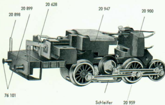
Fig. 4 Treibgestell (Beschwerung)
