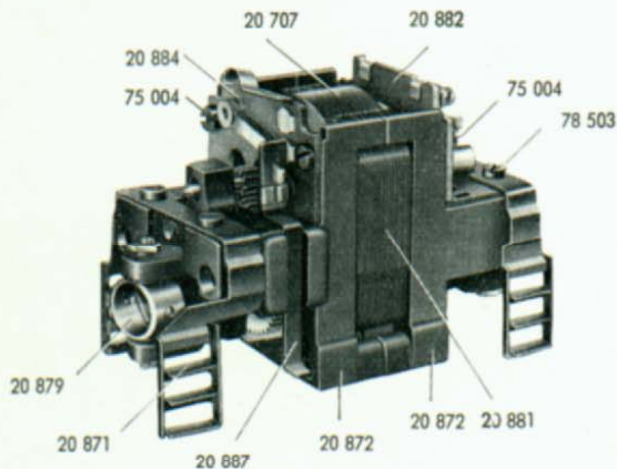
Fig. 3 Getriebemotor
