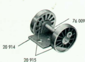
Fig. 7a Glatte Treibachse
