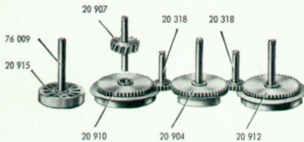
Fig. 7 Treibräder mit Gestänge
